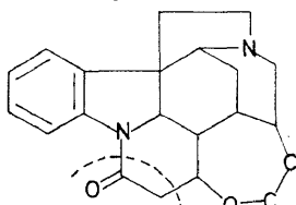
Strychnine
