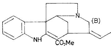
Akummicine
