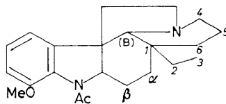
Aspidospermine
